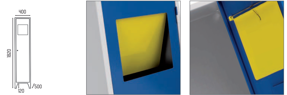
armários lavandaria
