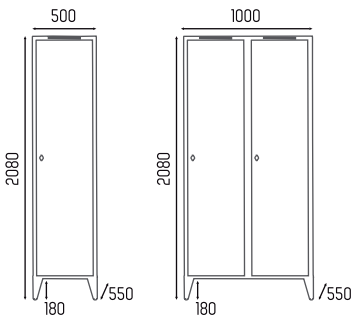
armários bombeiros
