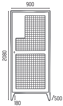
armários mergulhadores
