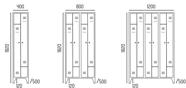
armários L
