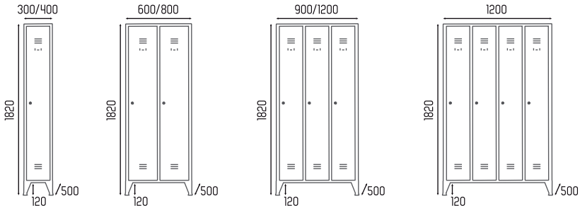
armários simples
